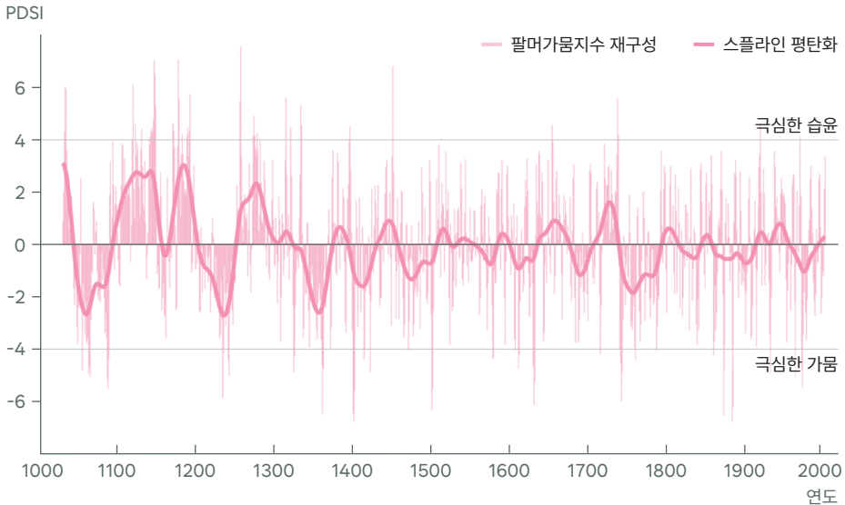
베트남 남부의 강수량 비도웁누이바국립공원(Bidoup Nui Ba National Park)의 편백나무 나이테 폭을 바탕으로 복원한 팔머가뭄지수(PDSI: Palmer Drought Severity Index)를 그래프로 나타낸 것이다.
