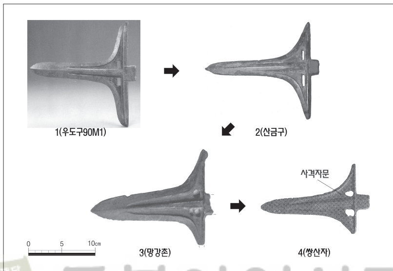
〈도면 9〉 요령식 동과의 변천
