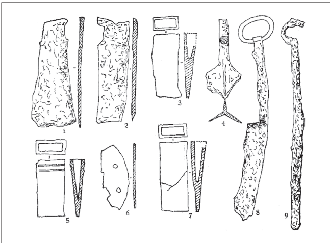
〈그림 4〉 철령 구태 철기
