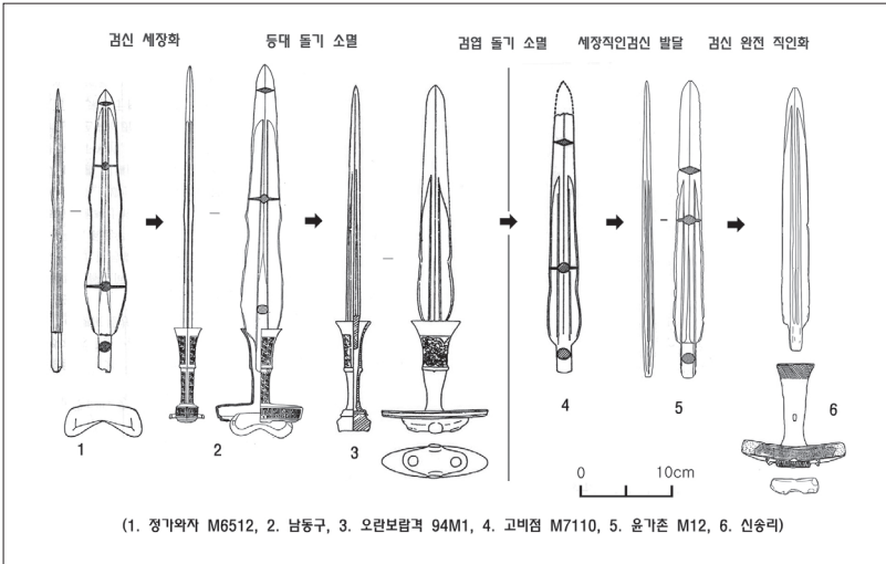
〈도면 6〉 윤가촌류 동검의 성립과 변천
